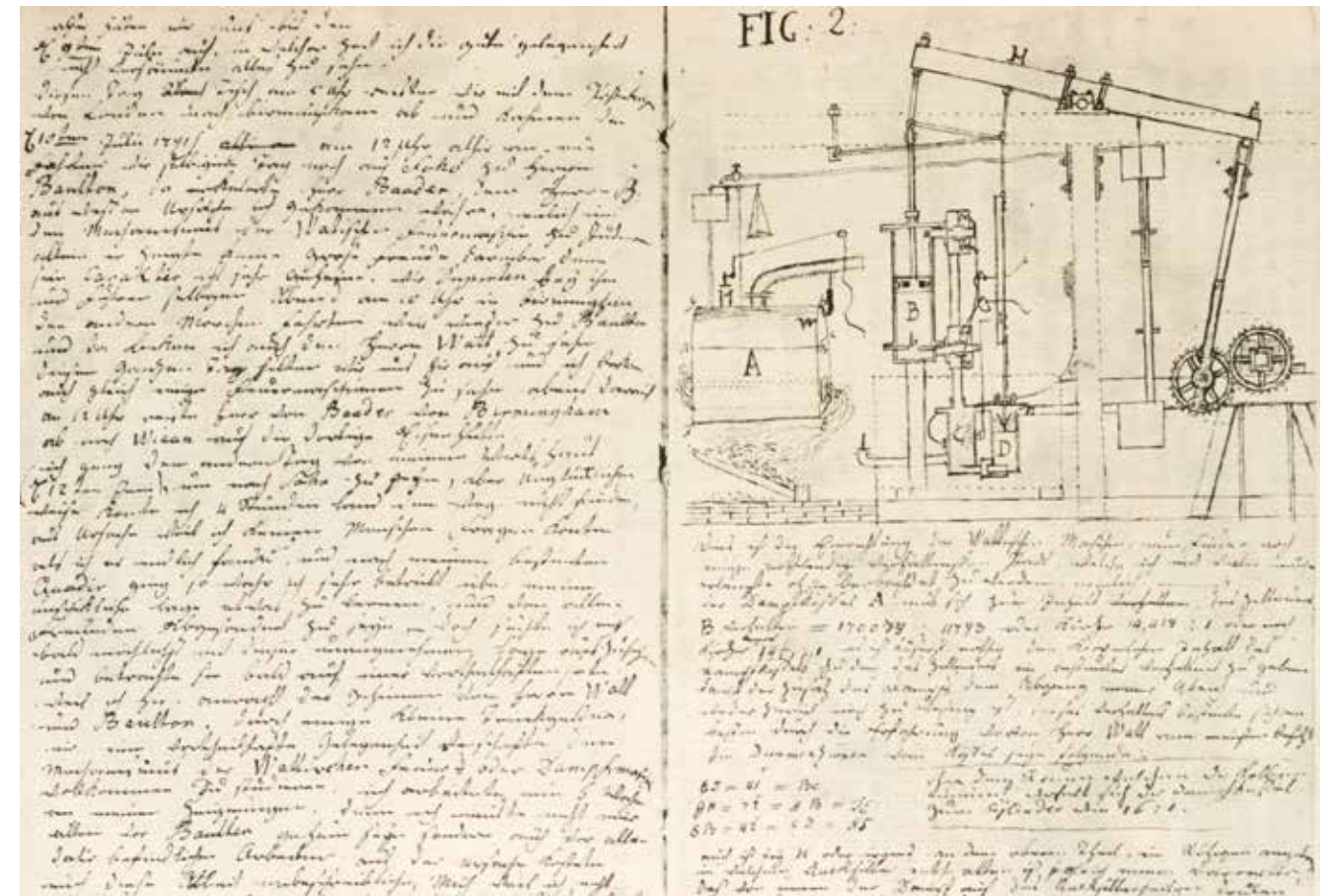
Zeichnung der Watt'schen Dampfmaschine, aus dem Tagebuch des Georg Friedrich von Reichenbach, 1791 (München, Deutsches Museum, Bibliothek)
